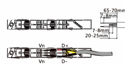
B. 顶部接线 配CX-9009
